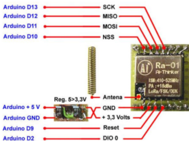
Figura 2. Conexiones del módulo Lora ra-01.
